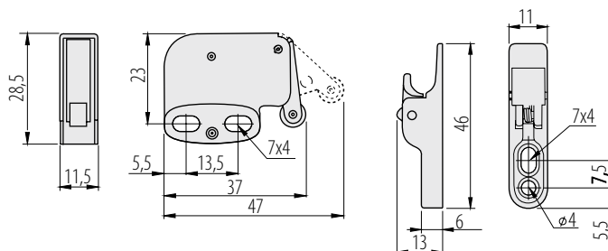
Wymiary montażowe / Mounting dimensions / Монтажные размеры
