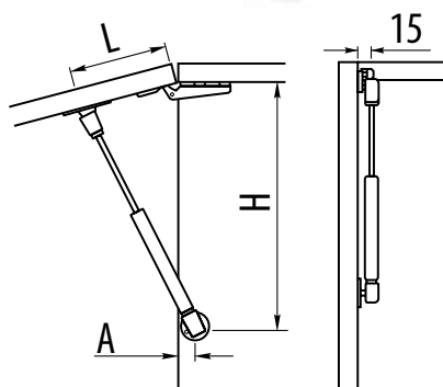
Drzwi wpuszczane / Flush door / Внутренние двери
