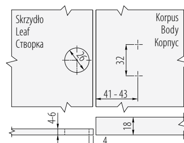
Drzwi zamknięte/ Door closed/ Закрытые дверцы
