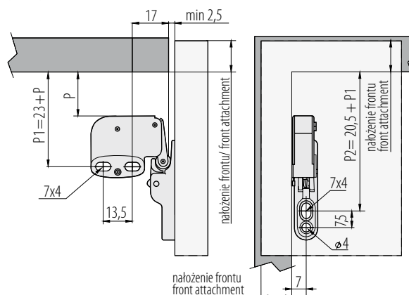
Wymiary montażowe / Mounting dimensions / Монтажные размеры
